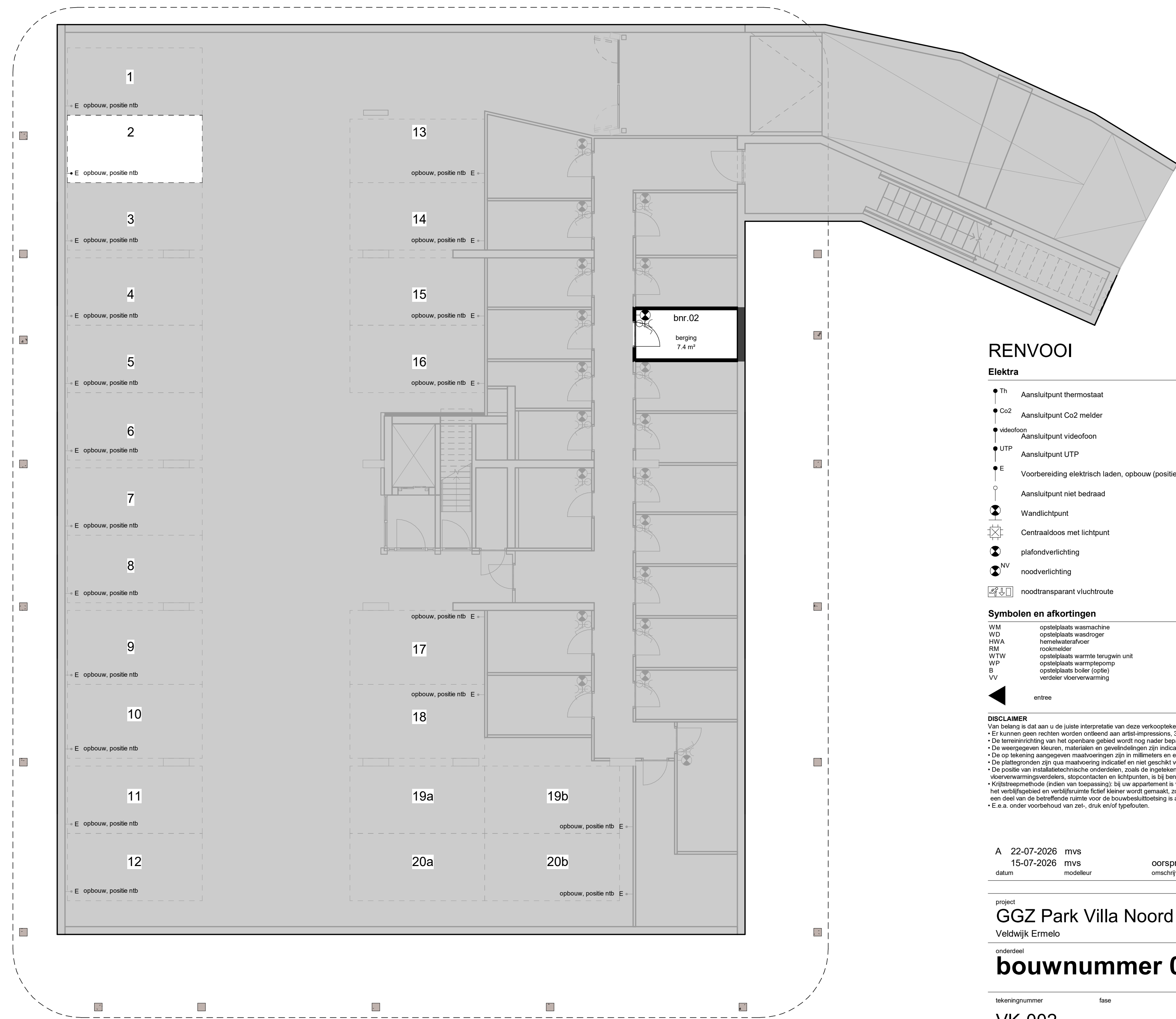
kelder - bouwnummer 02 1 : 100
