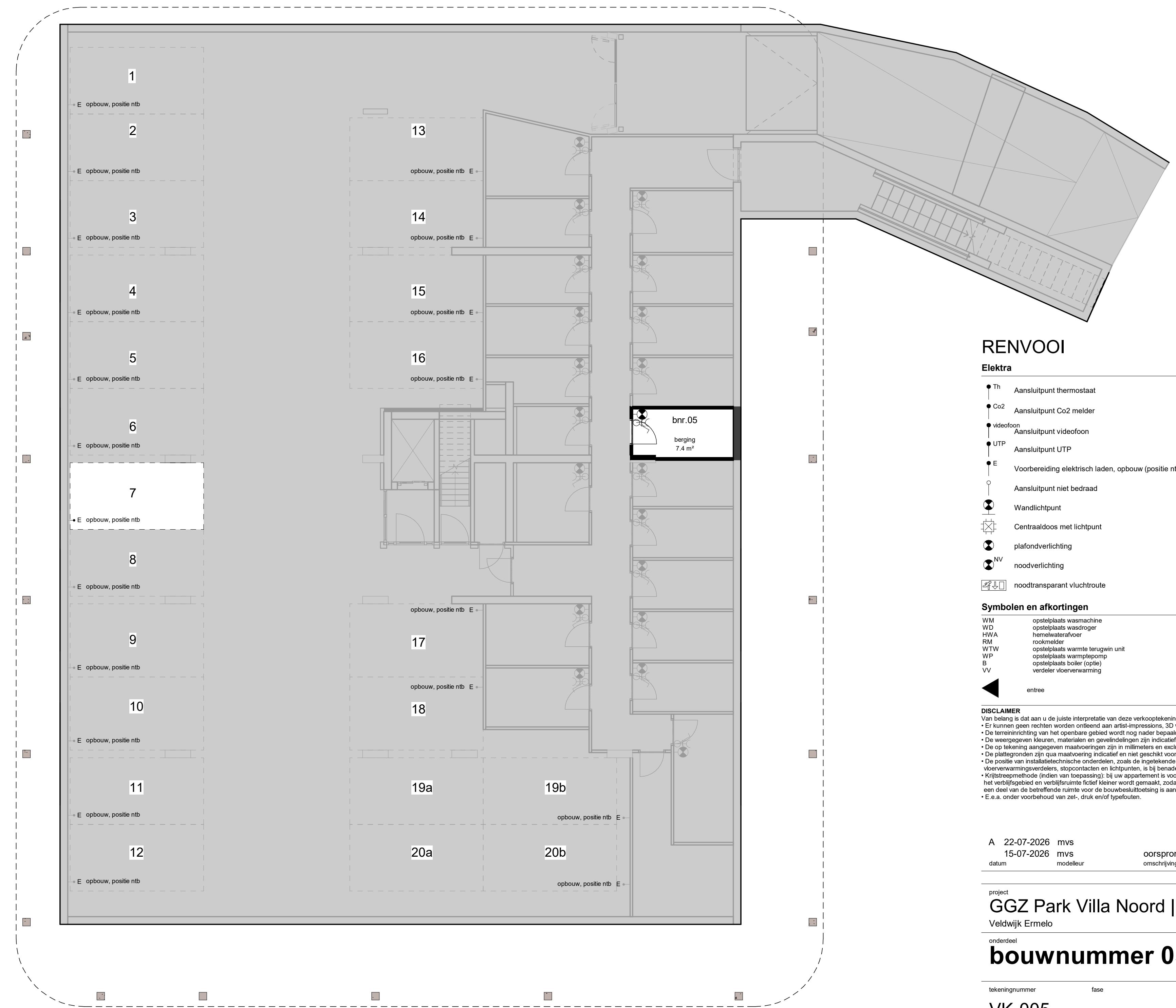
kelder - bouwnummer 05 1 : 100
