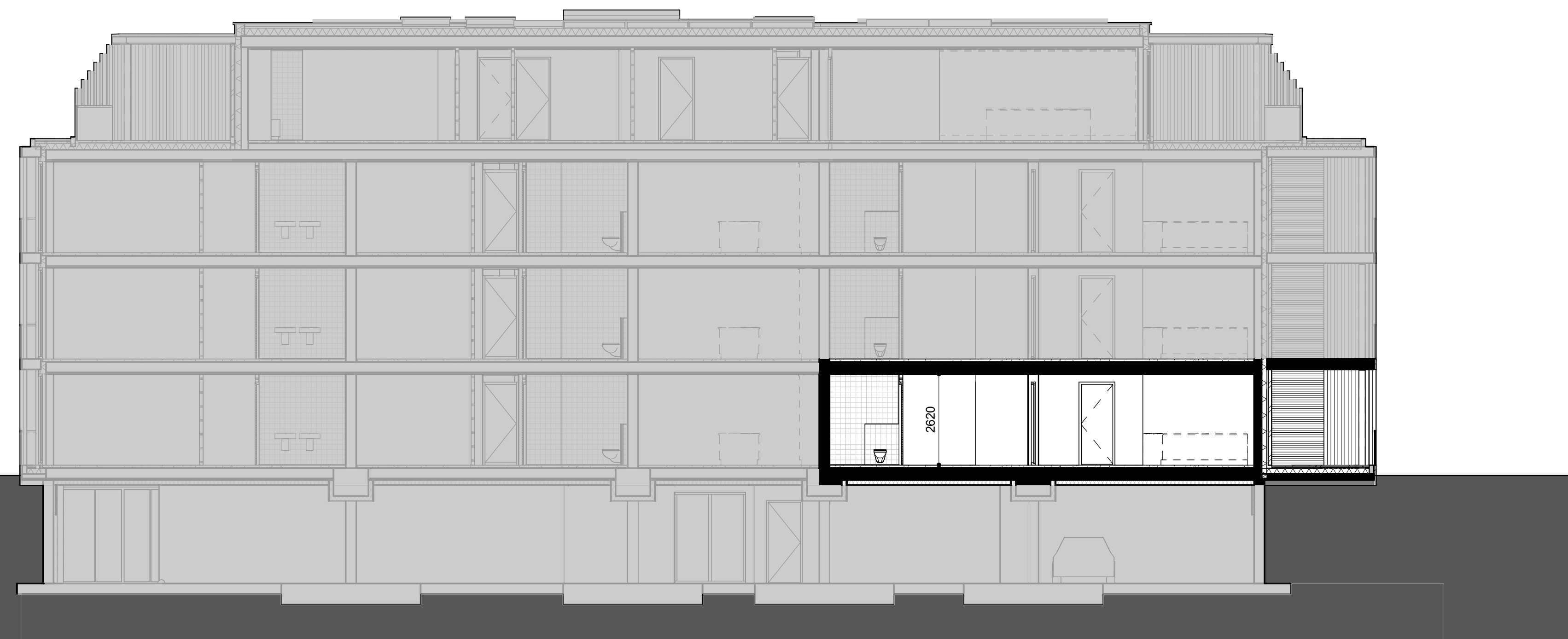
doorsnede - bouwnummer 05 1 : 100
