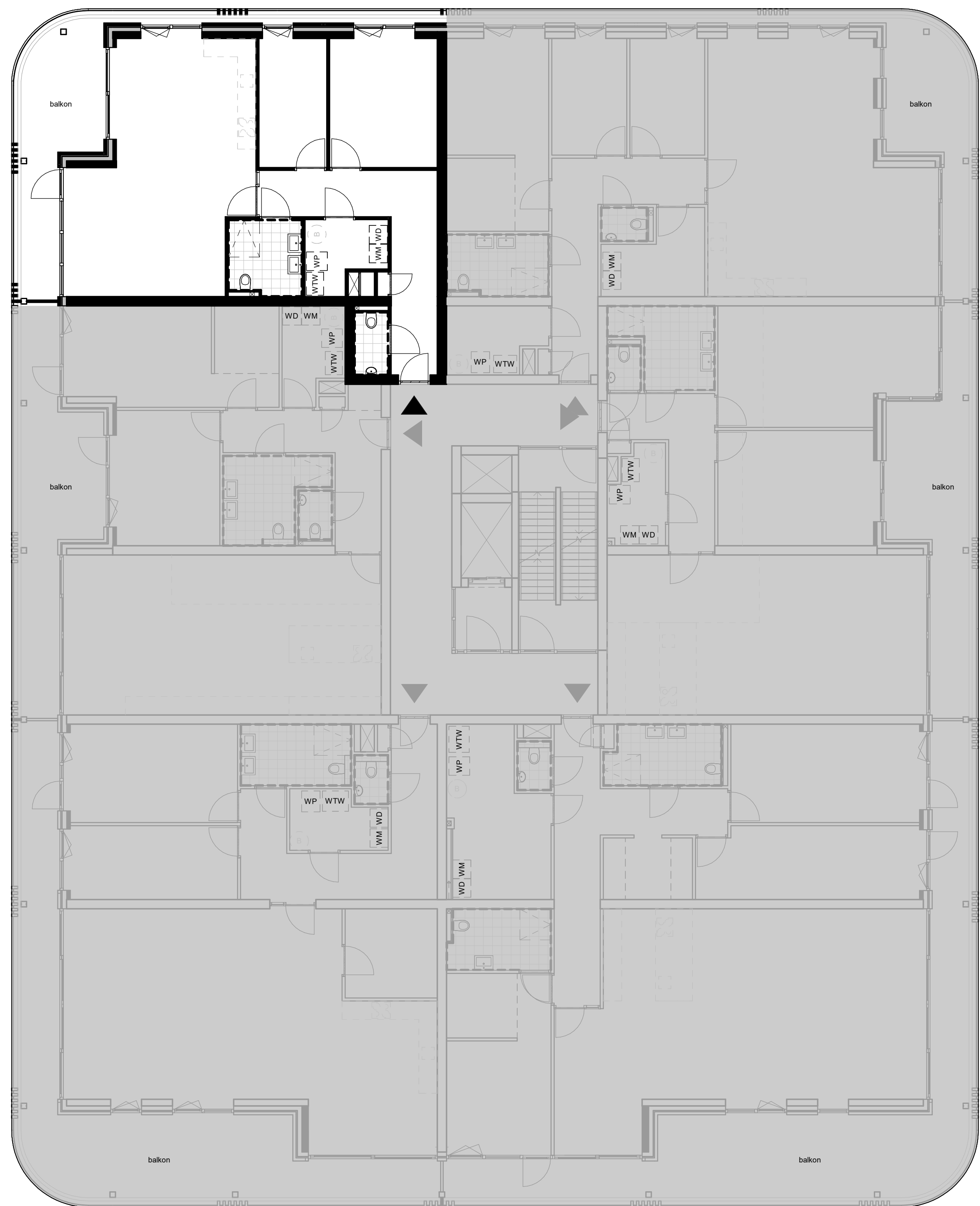
1e verdieping - bouwnummer 07 1 : 100
