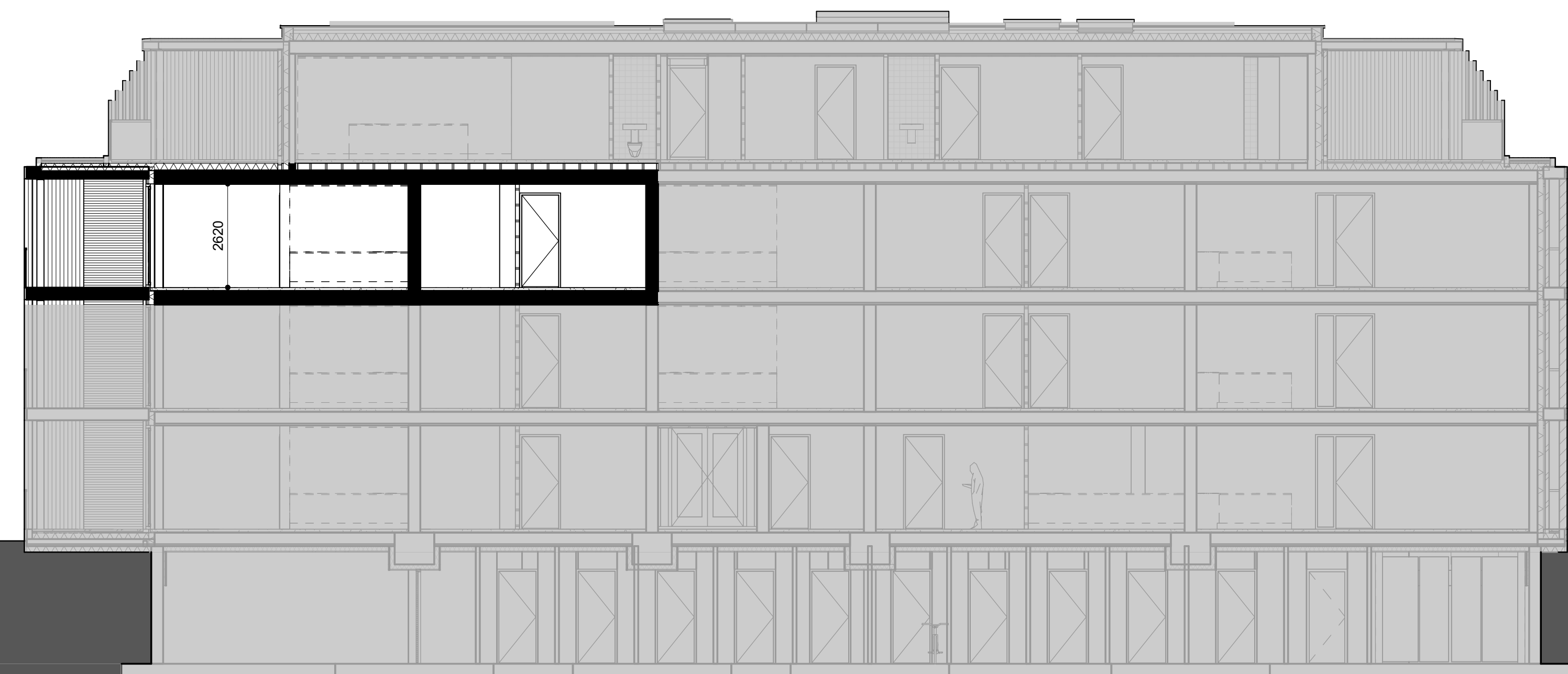
doorsnede - bouwnummer 16
